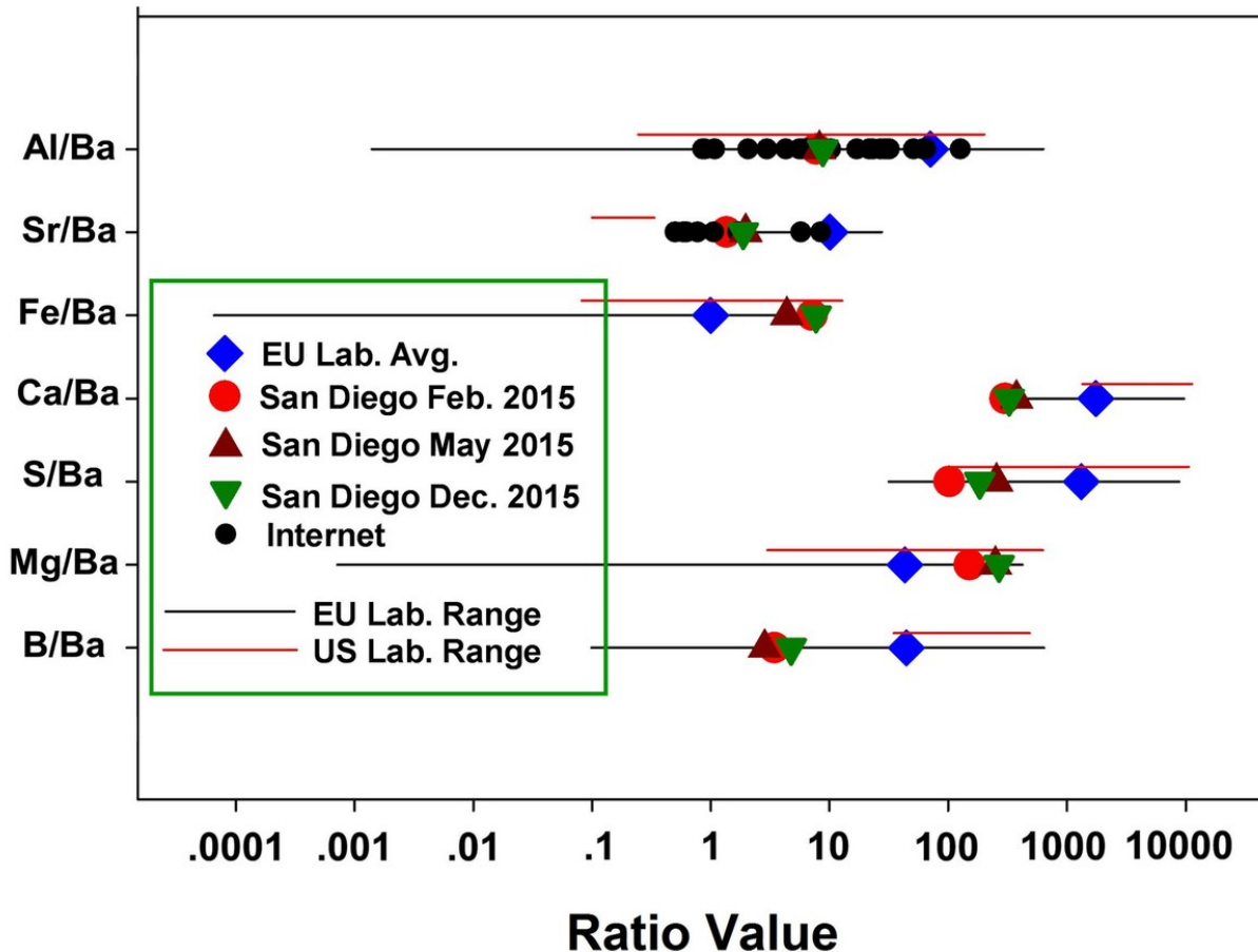
Figure 4. Analyse des ratios d'éléments dans les échantillons d'eau de pluie de San Diego collectés en février, mai et décembre 2015, présentés pour comparaison avec l'étendue des ratios correspondants des éléments et des valeurs moyennes de 23 lixiviats en laboratoire de cendres volantes de charbon européen (48) et 12 lixiviats de cendres volantes de charbon américain (55). Les ratios sur Internet publiés précédemment (14) d'éléments dans l'eau de pluie Al / Ba et Sr / Ba sont présentés à titre de comparaison.
