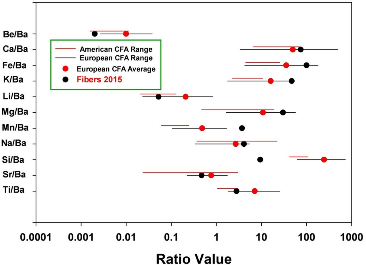
Figure 6 : Photographies de mailles fibreuses observées sur l'herbe après la fonte de la neige, montrant sa nature collante. Photos de Robest West avec sa permission. Figure 7 : 11 des 22 ratios d'éléments analysés de mailles fibreuses après la fonte de la neige, comparés aux ratios et moyennes des 23 échantillons de cendres volantes de charbon européen et de 12 échantillons de cendres volantes de charbon américain.
