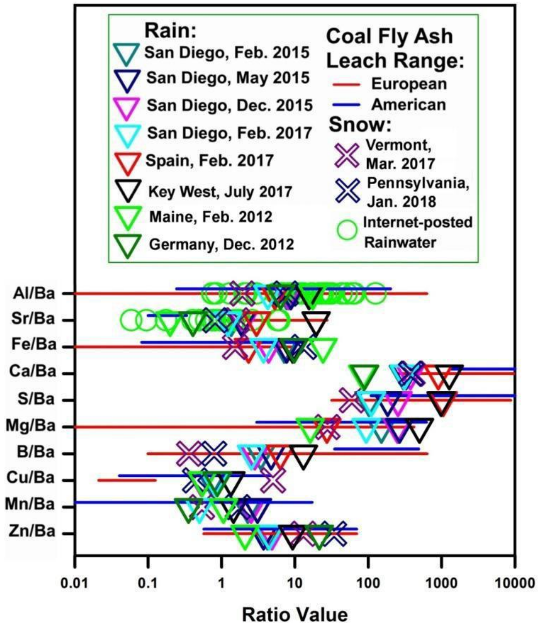
Fig. 5. Ratios d'éléments déterminés dans les échantillons d'eau de pluie et de neige collectés après pulvérisation aérienne. Les données de neige 2018 sont nouvelles; d'autres résultats ont déjà été rapportés [26,27]. Les lignes rouges et les lignes bleues, respectivement, sont des gammes d'expériences de lixiviation européennes [36] et américaines [38] des CVC.
