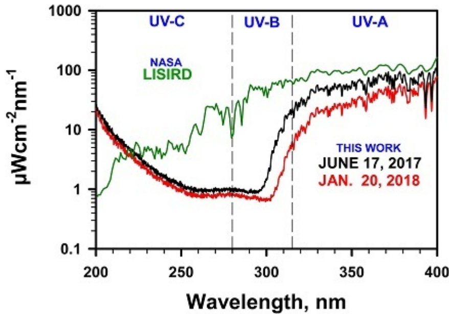
Fig. 6. Comparaison de notre irradiance spectrale solaire UV avec l'irradiance spectrale solaire dérivée du satellite LISIRD de la NASA au sommet de l'atmosphère [31]
