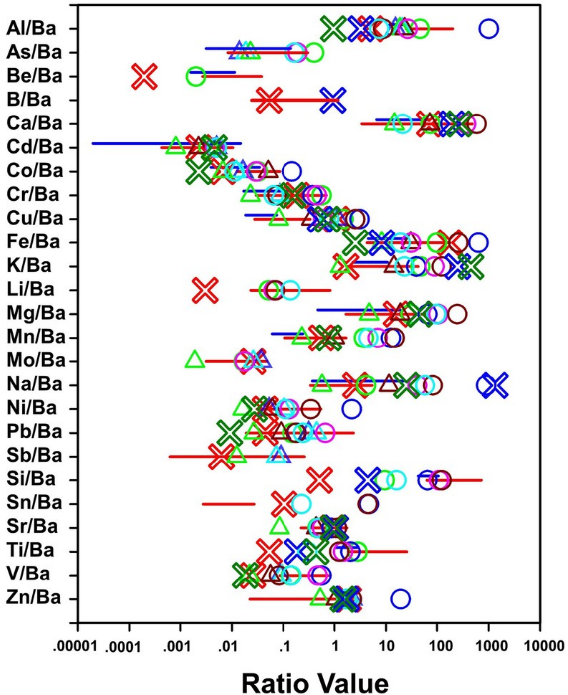
Fig. 4 Ratios en éléments chimiques, mesurés sur les échantillons de substance tombée indiqués par les symboles X: vert : département de la qualité environnementale du Michigan, rouge : Northern Lake Service et bleu : Basic Laboratory. À titre de comparaison, les lignes rouges et bleues sont respectivement les proportions des éléments mesurés sur des échantillons de cendres volantes européennes [25] et américaines [26] ; les cercles sont des ratios en éléments des échantillons de fibres ( Fig.5) trouvés sur l'herbe à la fonte de la neige à Laona, Wisconsin (USA) le 19 mars 2015, et les triangles sont les ratios en éléments mesurés sur la poussière recueillie sur les filtres à air extérieurs, de haute qualité, par périodes de trois mois [13,23].
