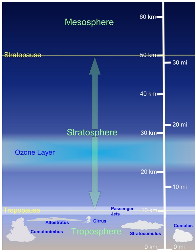
Figure 1. Représentation schématisique des couches de l'atmosphère à latitudes moyennes montrant les régions typiques de formations de nuages et la circulation des avions de passagers.
