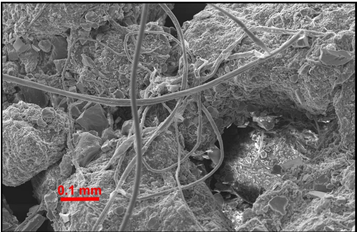
Fig. 10 Image au microscope à balayage électronique de cryoconite de la banquise du Groenland montrant un réseau de filaments cyanobactériens autour des fragments minéraux (photo de Joseph Cook, avec son aimable autorisation).
