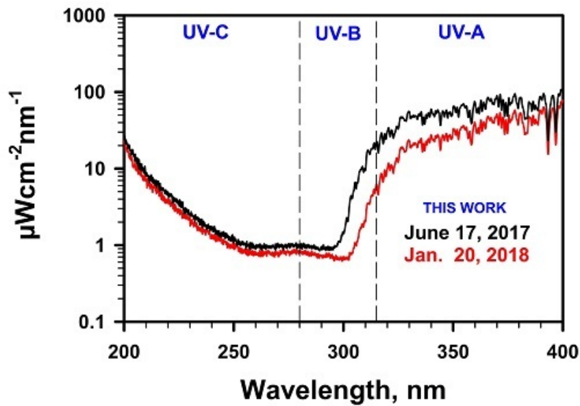
Fig. 3. Exemples de nos mesures d'irradiance spectrale solaire
